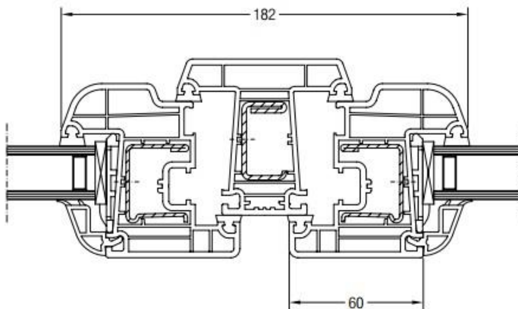
Sezione nodo anta arrotondata
