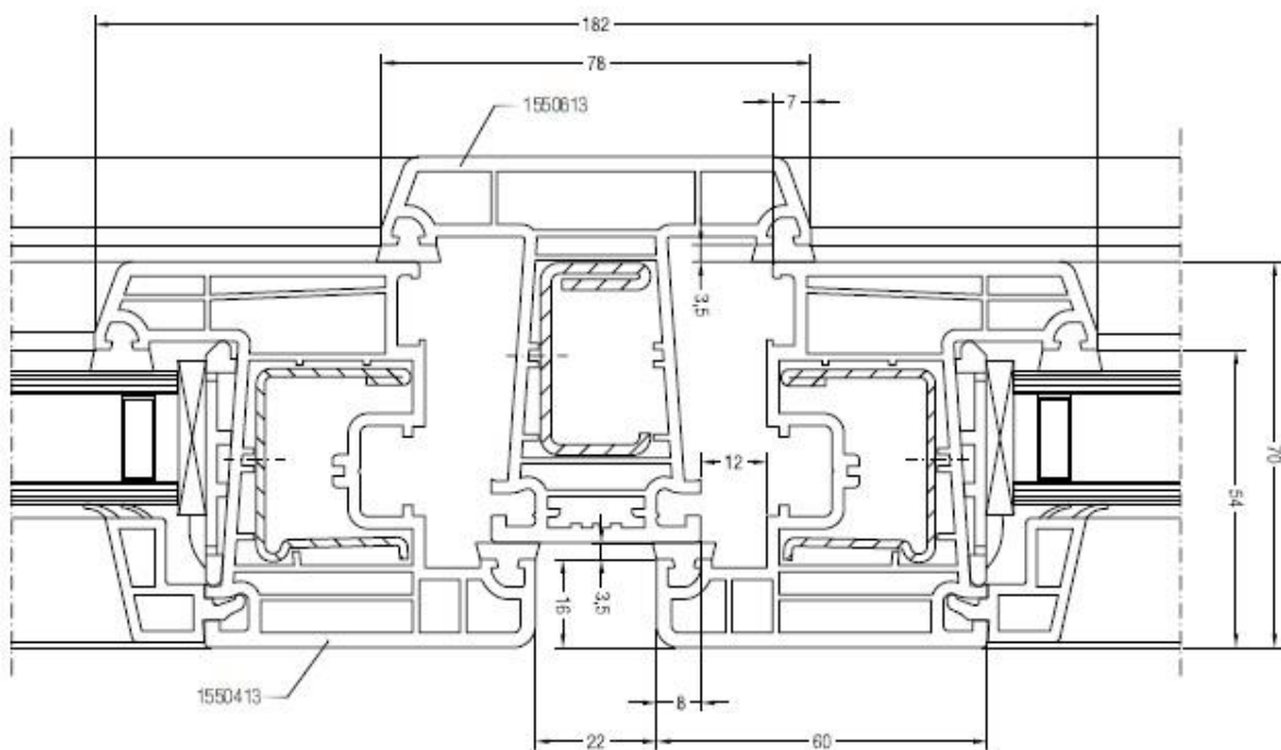
Sezione nodo anta dritta
